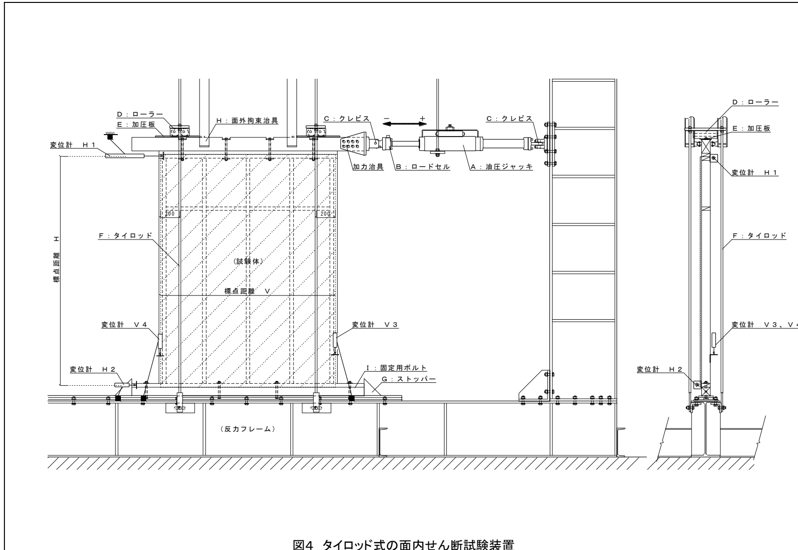
図4 タイロッド式の面内せん断試験装置
