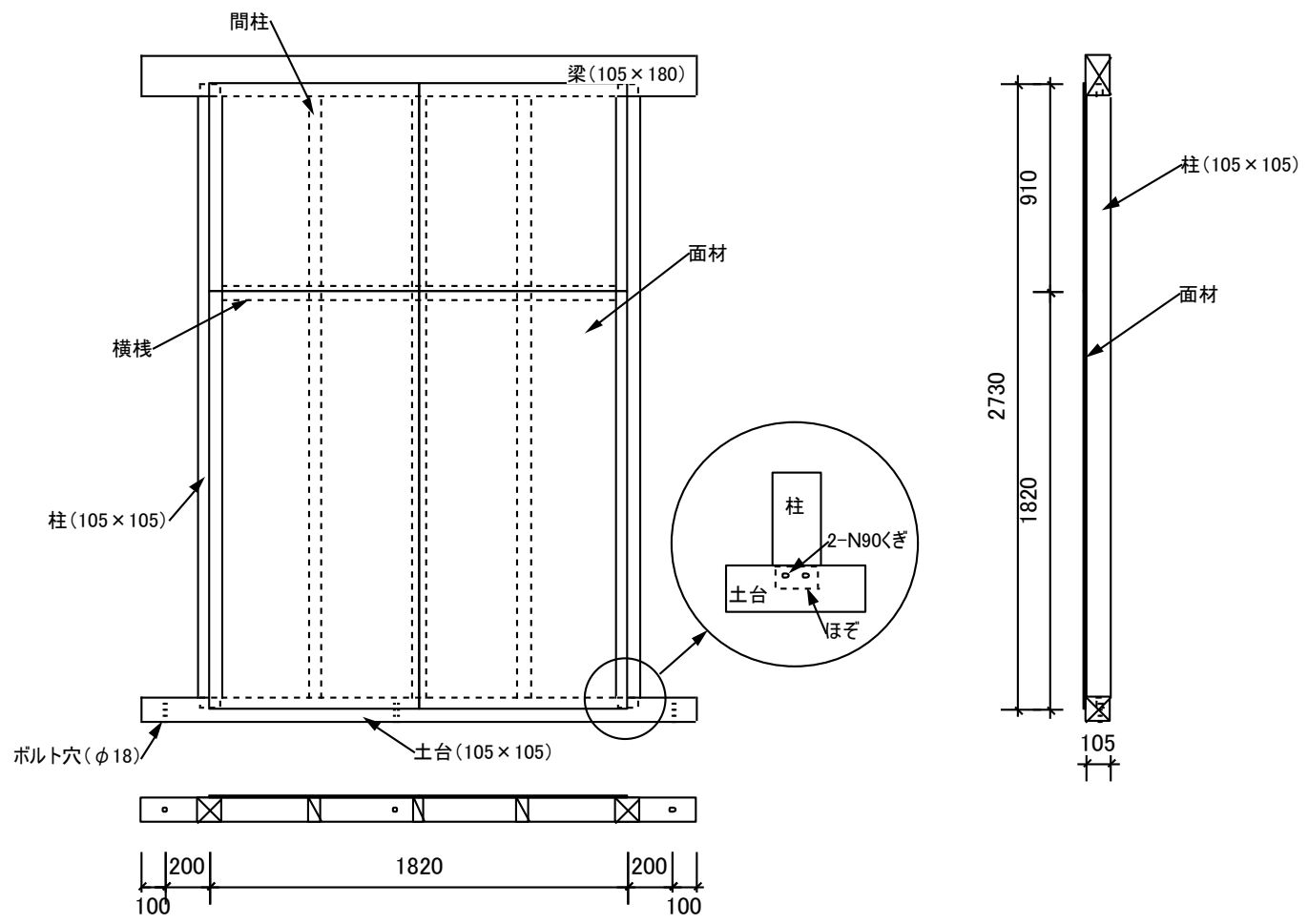
図1 軸組耐力壁の試験体例(面材系)単位:mm
